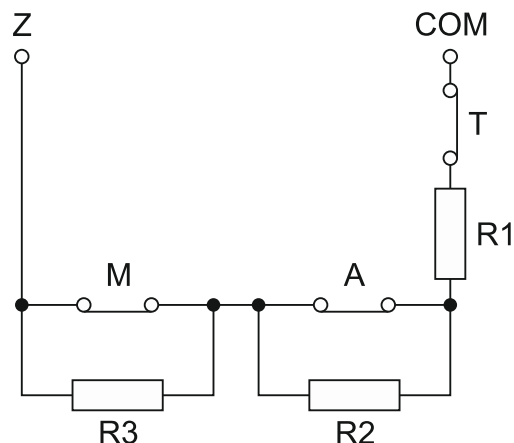
Рис. 4. Нумерация оконечных резисторов. Т – тампер. А – тревога. М – экранирование. В случае шлейфов EOL и 2EOL значение резистора R3 не имеет значения. В случае шлейфов EOL значение резистора – это сумма значений, запрограммированных для резисторов R1 и R2.
