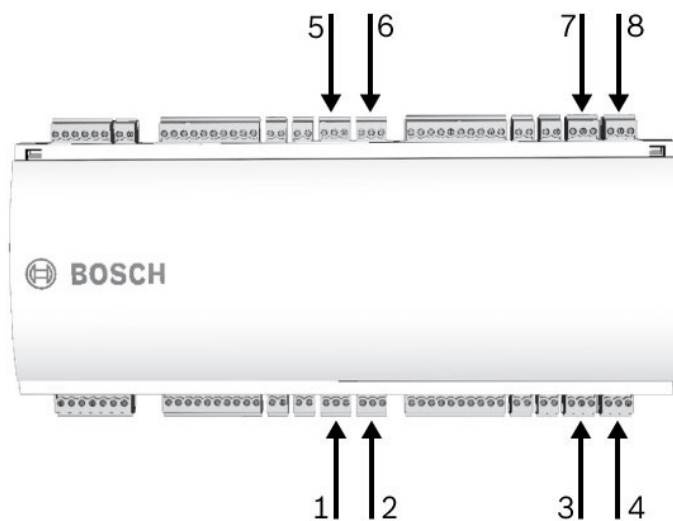
Рис. 4.12: Расположение разъемов релейных выходов
