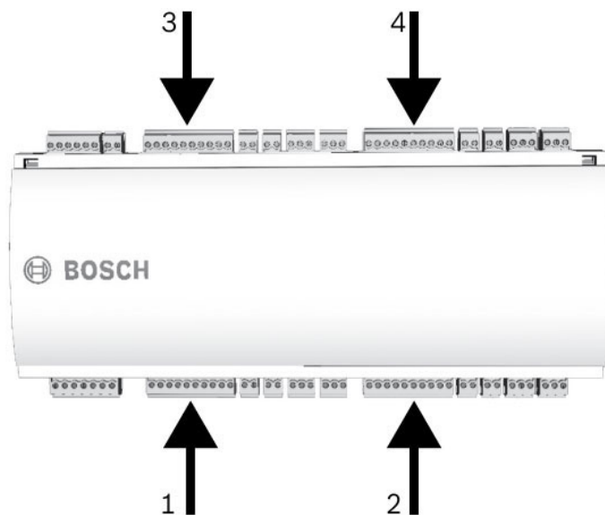
Рис. 4.11: Расположение интерфейсов Wiegand для внешних устройств
