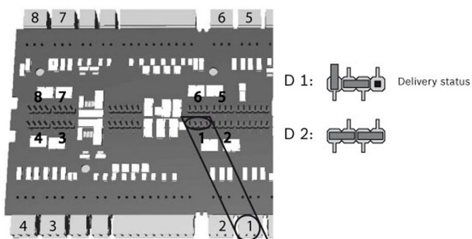
Рис. 4.13: Расположение перемычек релейных выходов (нижняя сторона)
