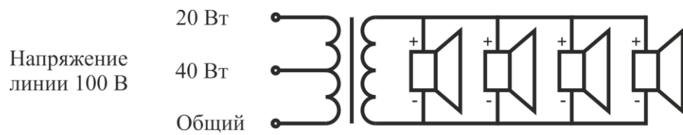
Рис. 2. Схема подключения оповещателя.
