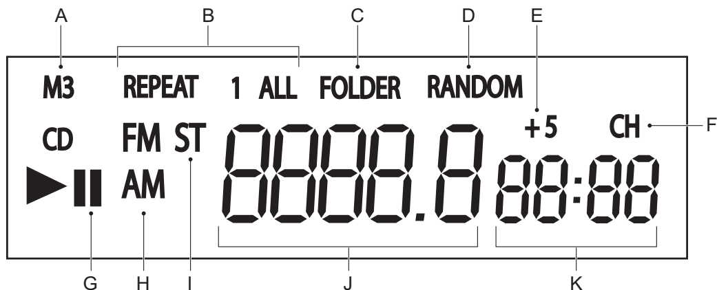
Рисунок 8.4: ЖК-дисплей (1) SD/USB/ПРИЕМНИК
