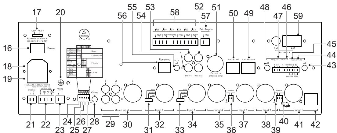
Рисунок 6.1: Задняя панель
